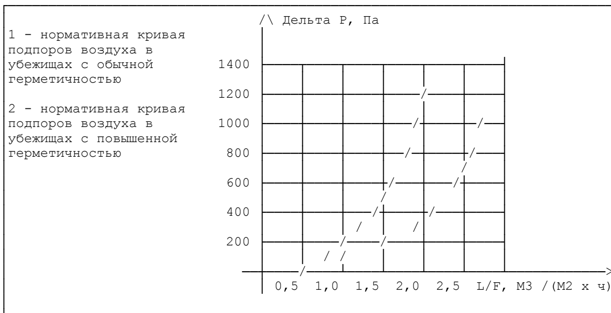
ГРАФИК ДЛЯ ОЦЕНКИ ГЕРМЕТИЧНОСТИ УБЕЖИЩ
